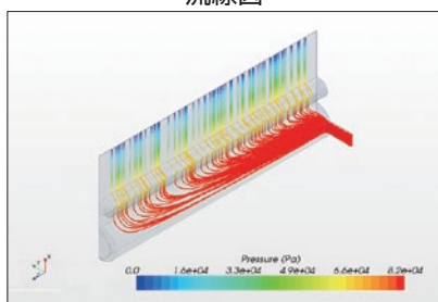
流線図
