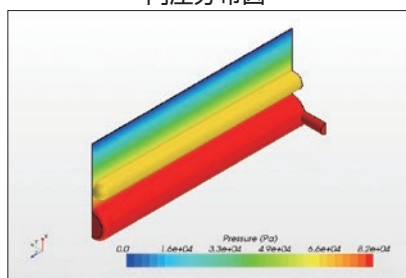
内圧分布図
